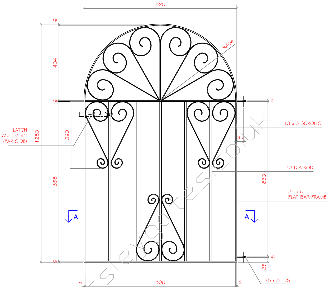
ELEVATION
